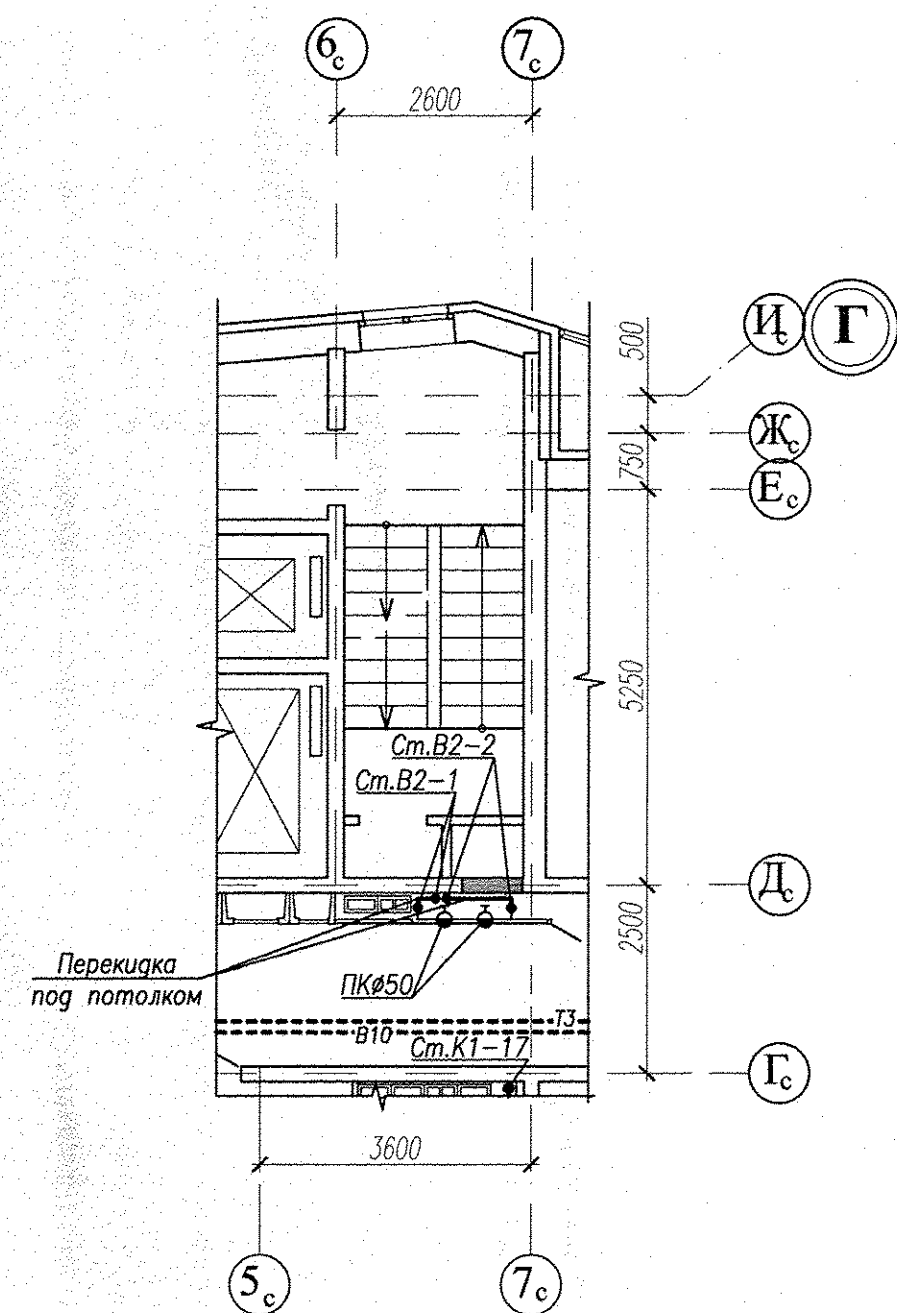
Фрагмент плана 16 этажа в 17-этажной секции
